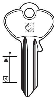
HEAD TYPE / TESTA TIPO F
